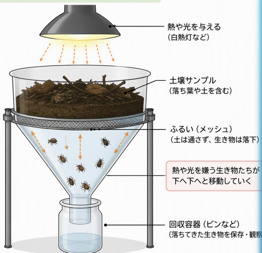
ツルグレン装置の模式図
